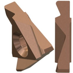
On Edge Grooving
